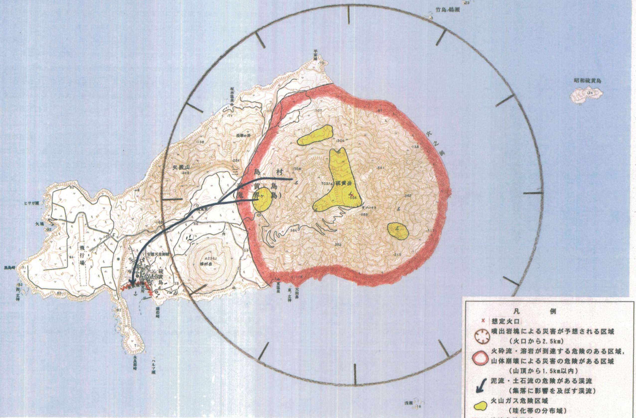
図5-2-3 薩摩硫黄島火山災害危険区域予測図
